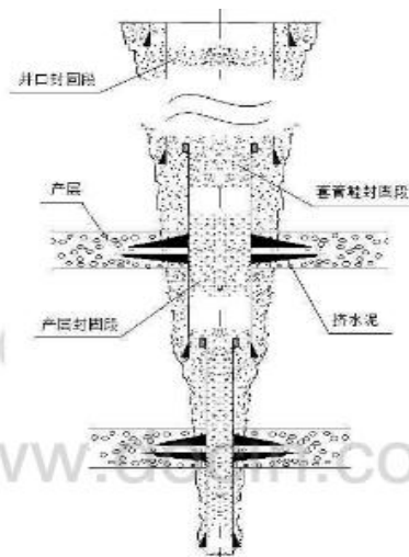
图 8 永久封井结构示意图
