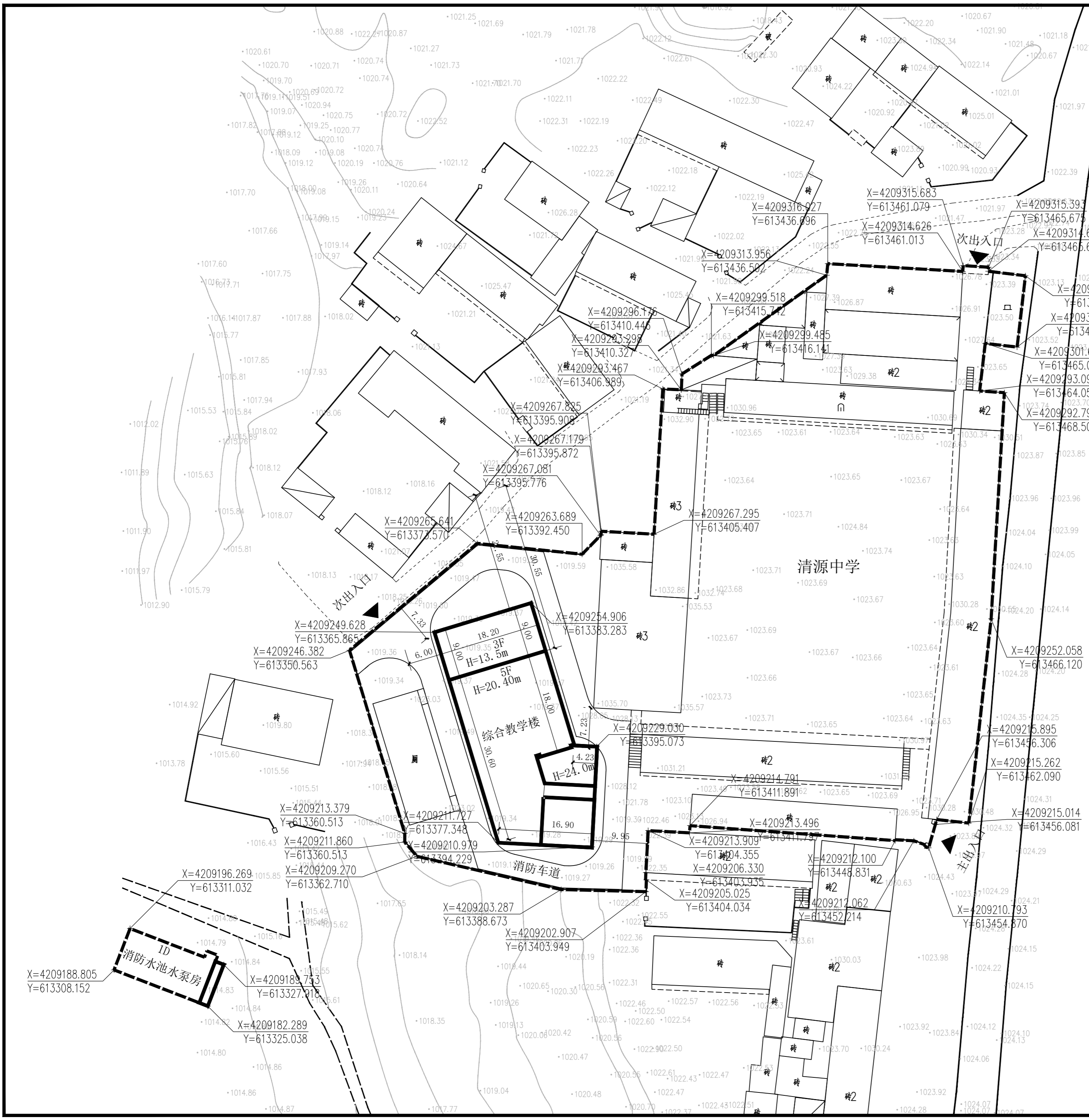
总平面布置图 1:500
