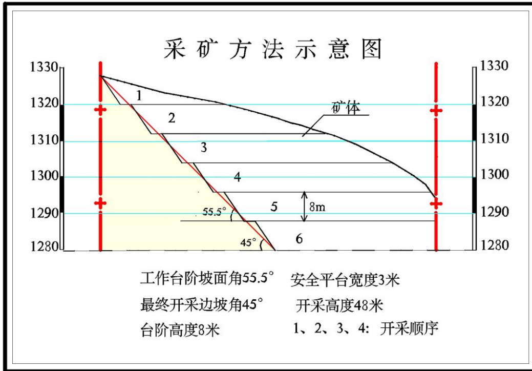
图 1.3-2 鼎盛砖厂采矿方法示意图
