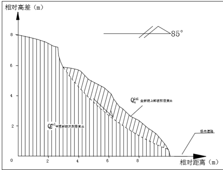
图 3.2-1 H1 滑坡隐患剖面图
