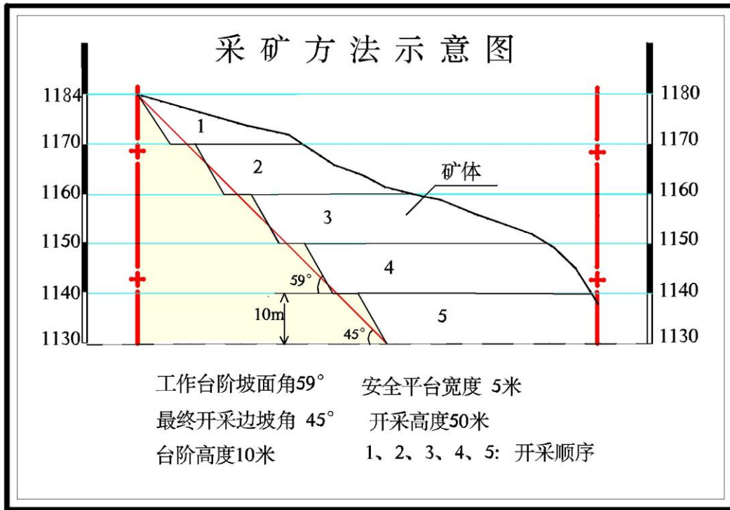
图 1.3-2 振兴砖厂采矿方法示意图
